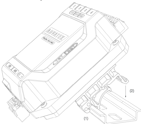
Figure 4 : Contrôleur fixé à un rail DIN
