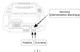
Figure 1 : Emplacement de l'alimentation électrique
