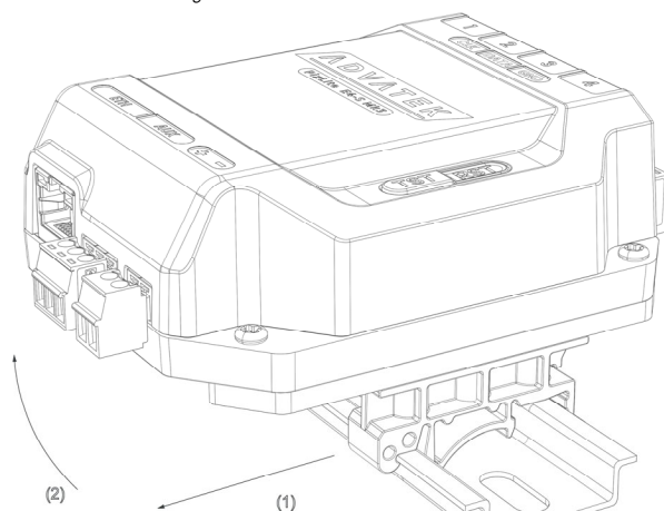
Figure 5 : Retrait d'un contrôleur du rail DIN
