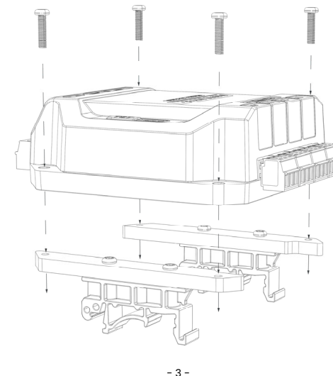
Figure 3 : Contrôleur fixé à un support
