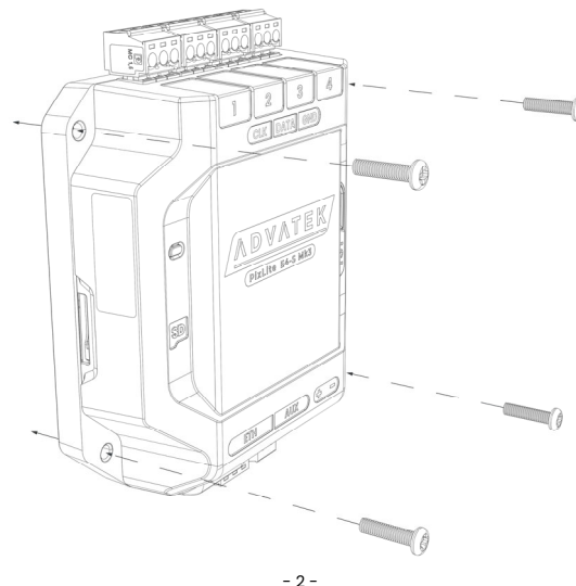
Figure 2 : Contrôleur fixé au mur
